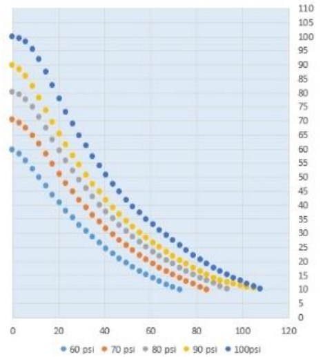
DESCARGA – CANHÃO 100 LITROS PRESSÃO(psi) X TEMPO(mseg)
